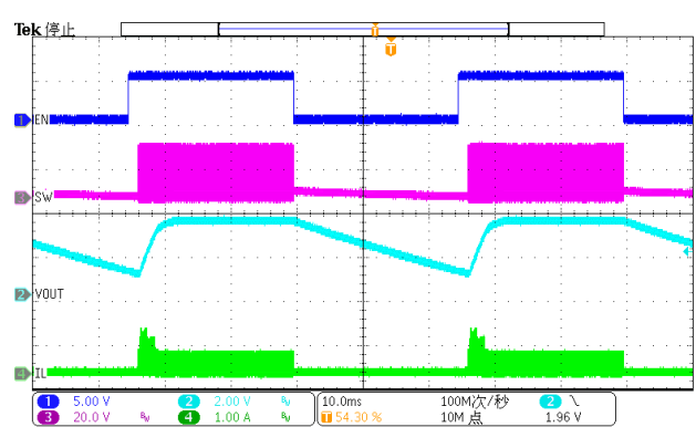
Figure 16. EN toggle (Iload=20mA)
